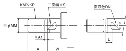
基準寸法表
