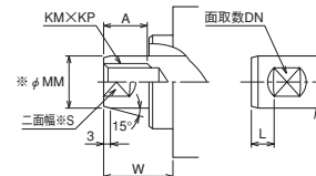
基準寸法表
