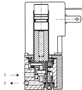
2/2 - NO
