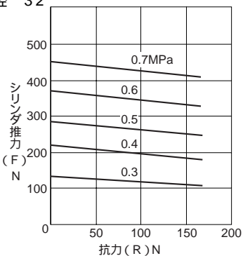
グラフ[A]-5 シリンダ推力 - 抗力関係図 内径 32
