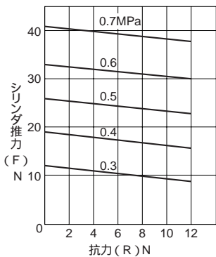
グラフ[A]-3 シリンダ推力 - 抗力関係図 内径 20
