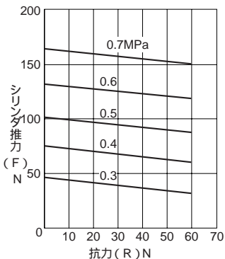
グラフ[A]-5 シリンダ推力 - 抗力関係図 内径 32
