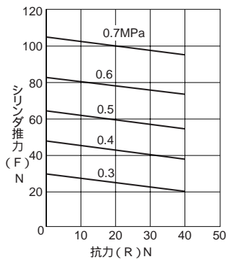
グラフ[A]-4 シリンダ推力 - 抗力関係図 内径 25
