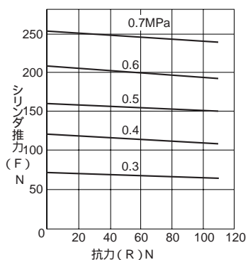
グラフ[A]-6 シリンダ推力 - 抗力関係図 内径 40
